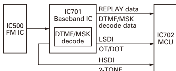
Fig. 15 Decode
