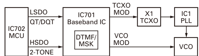
Fig. 14 Encode
